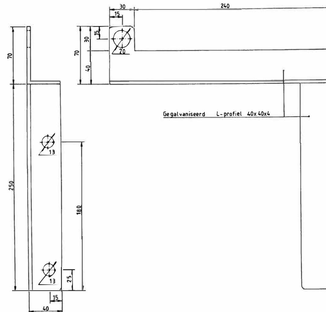
ZIJAAANZICHT
