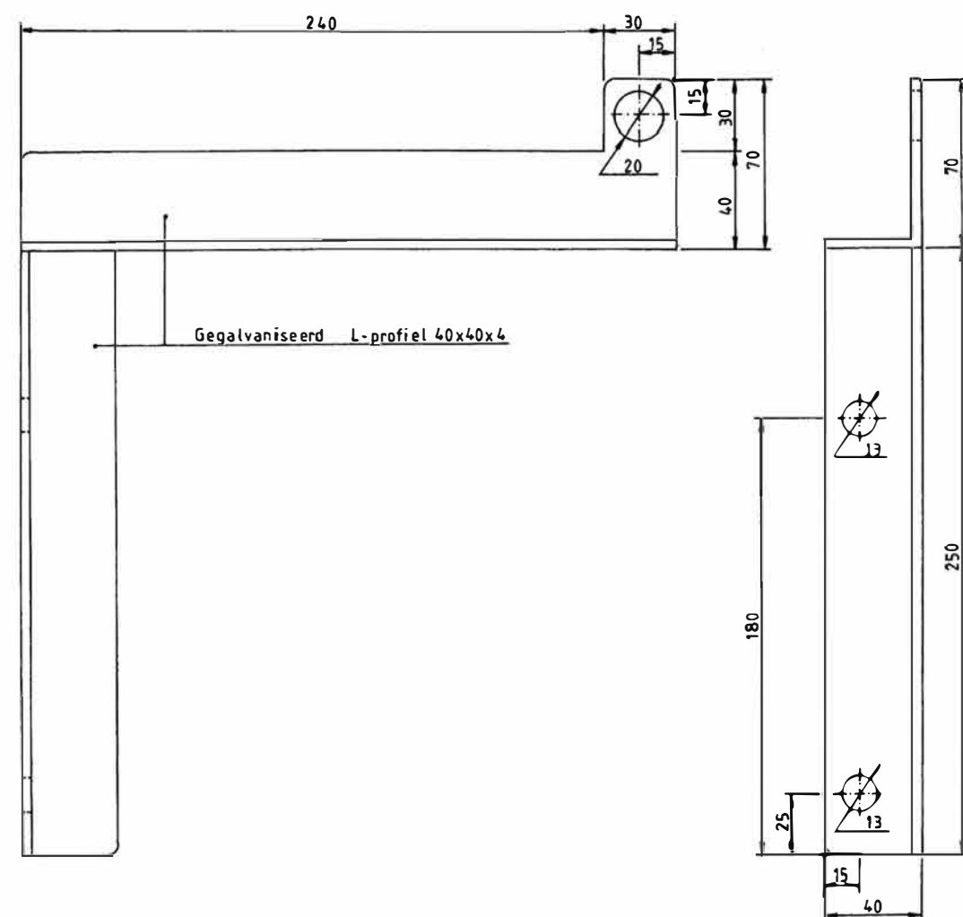
VOORAANZICHT
