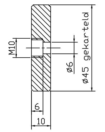
②b Handwiel
