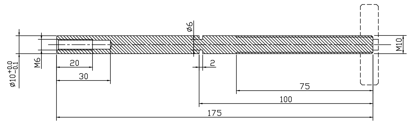
②a Binnenas
