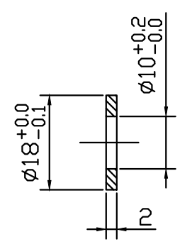
⑤ Sluitring
