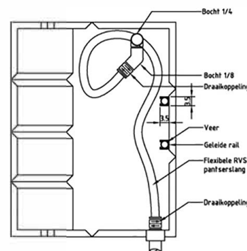
SNEDE D-D'
