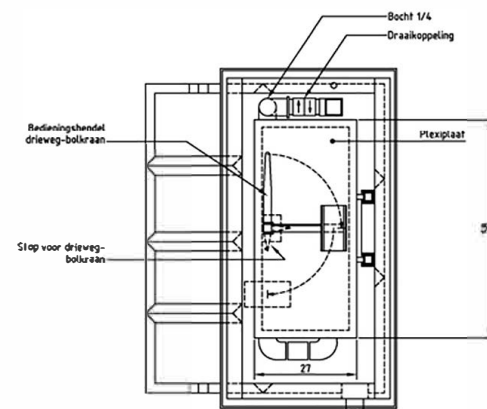
SNEDE B-B'
