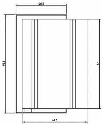
ONDERAANZICHT
