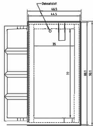
BOVENAANZICHT
