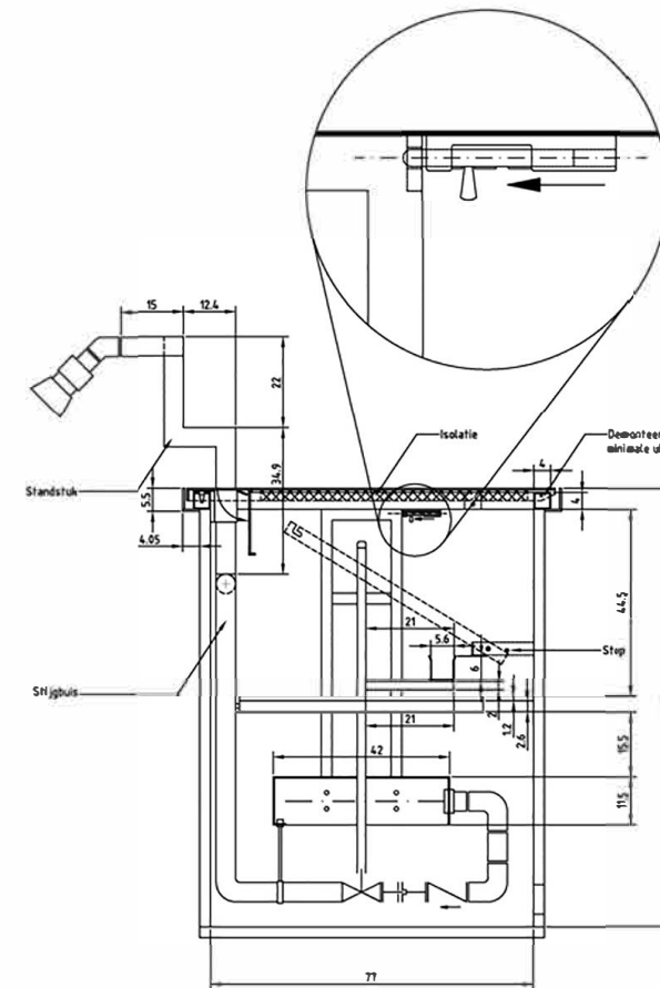
SNEDE A-A'
