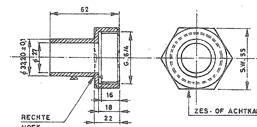
30 PASSTUK voor uitzettingsvoeg G.5/4
