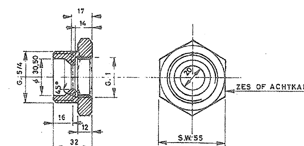
31 OVERGANGSSTUK G.5/4 (bu) - G.1 (bi)
