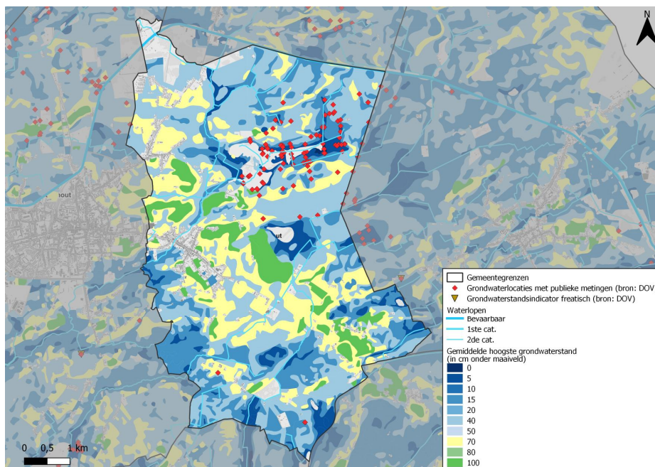
Figuur 2-2: Gemiddelde hoogste grondwaterstand (GHG), grondwaterlocaties met publieke metingen en locatie van de freatische grondwaterstandsindicator in Oud-Turnhout (DOV Vlaanderen, 2021).
