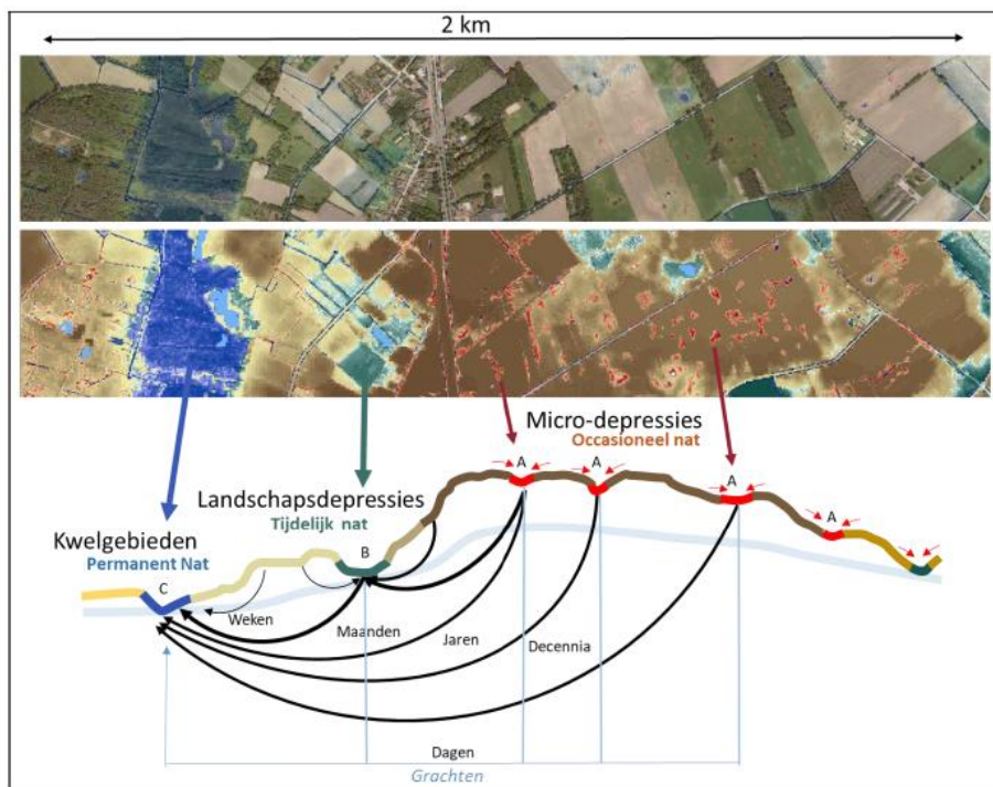
Figuur 3-1: Illustratie van de watersysteemkaart aan de hand van een doorsnede van het landschap. De verschillende zones op de watersysteemkaart houden verband met de positie in het landschap. Impliciet is dit gerelateerd aan de potentiële verblijftijd van het geïnfiltreerde water. Grachten verkorten de verblijftijd (Staes, 2021).
