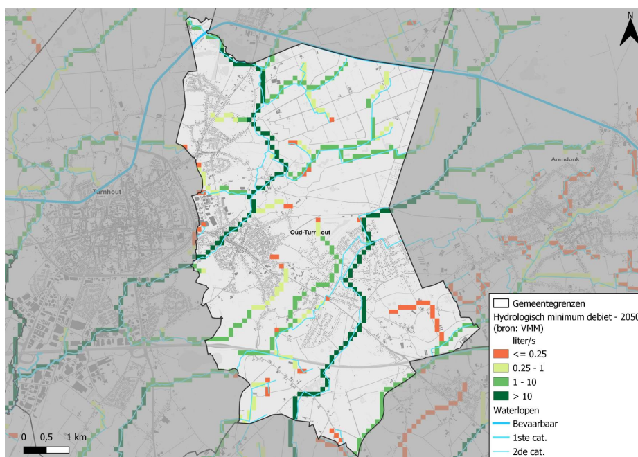
Figuur 2-8: Hydrologisch minimum debiet in waterlopen in Oud-Turnhout, bij een herhalingsperiode van 2 jaar; scenario 2050 (VMM, 2020).
