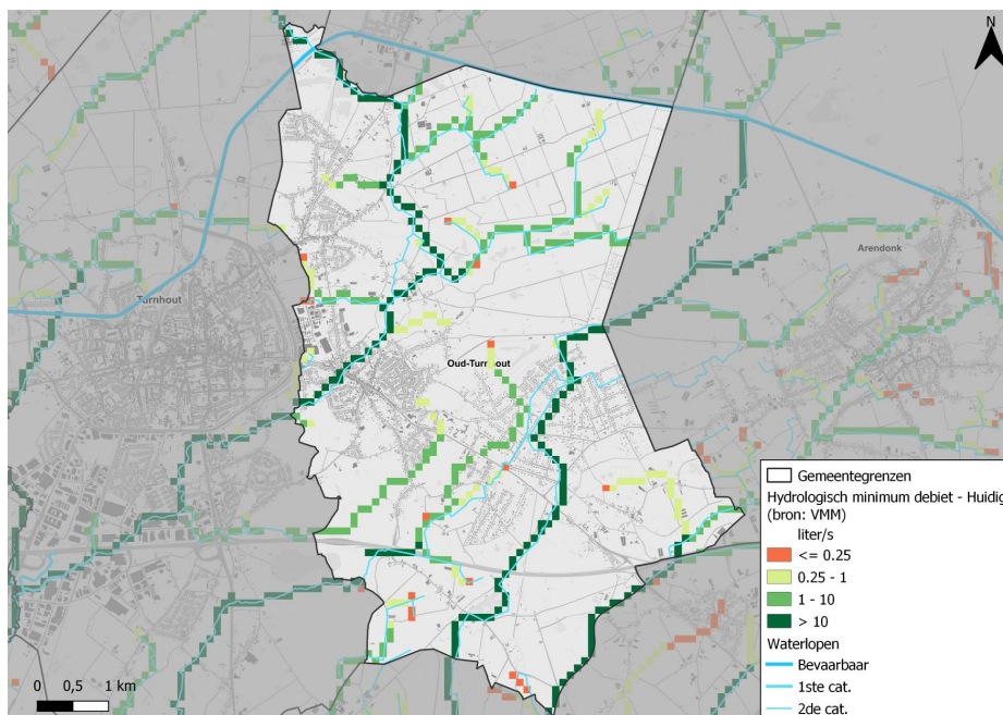
Figuur 2-7: Hydrologisch minimum debiet in waterlopen in Oud-Turnhout bij een herhalingsperiode van 2 jaar; huidige toestand (VMM, 2020)
