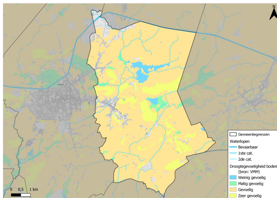
Figuur 2-4: Droogtegevoeligheid van de bodem in Oud-Turnhout; huidige toestand (VMM, 2020).
