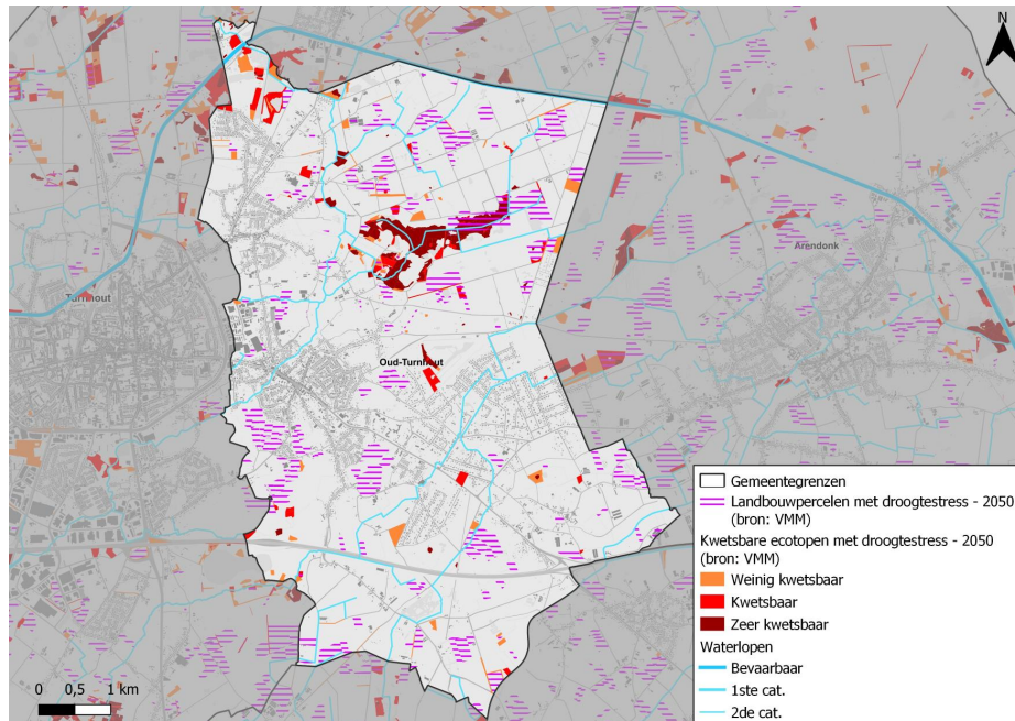
Figuur 2-6: Droogtegevoeligheid van landbouwpercelen en ecotopen in Oud-Turnhout; scenario 2050 (VMM, 2020)
